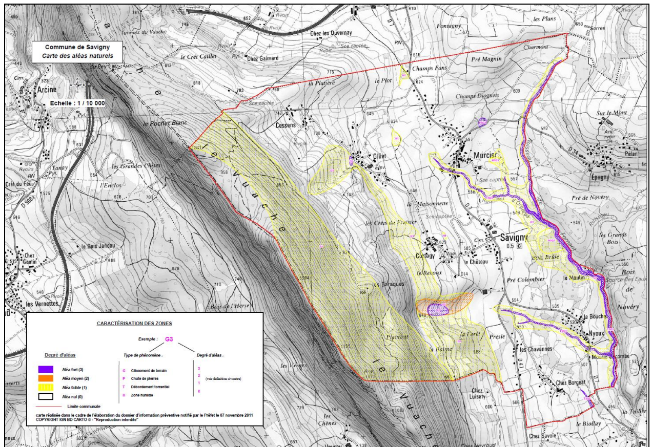
Fig. 2. Carte des aléas naturels – commune de Savigny
